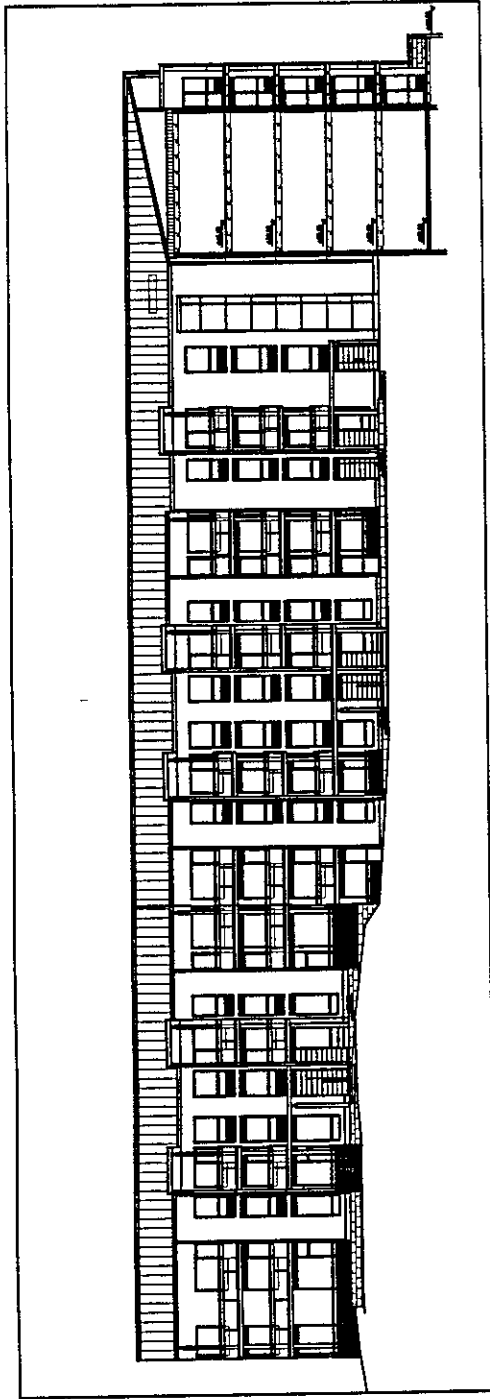
JULKISIVU LÄNTEEN
