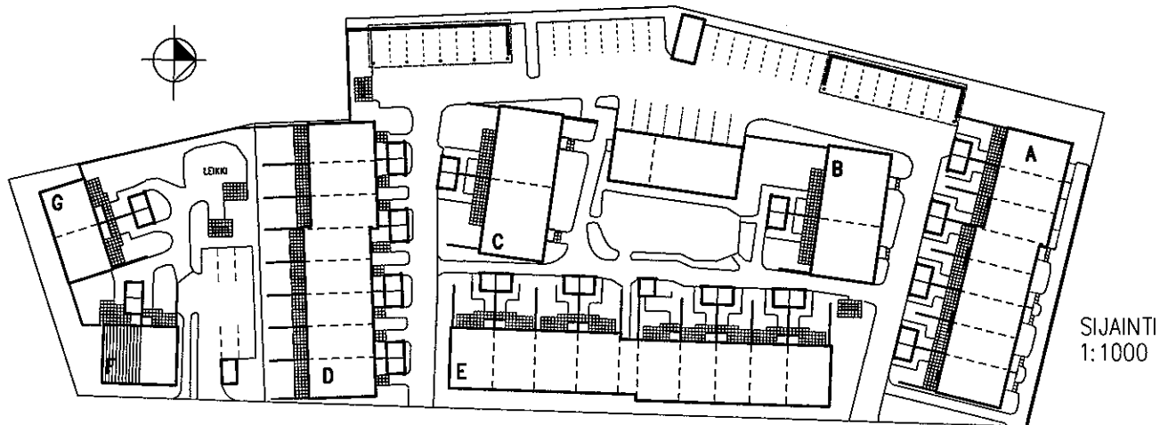
KUVERNÖÖRINTIE
