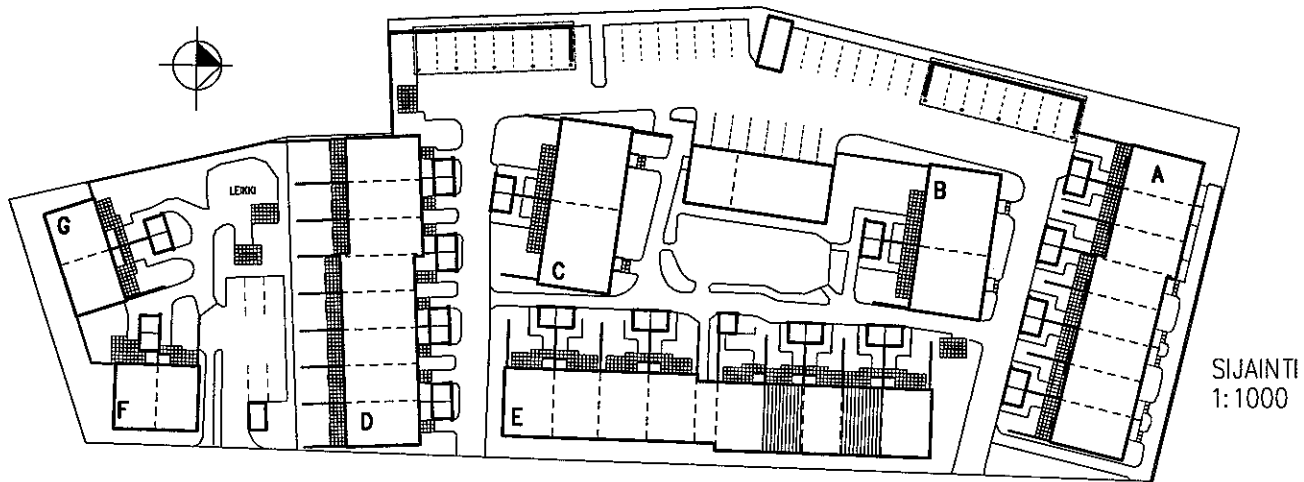
KUVERNÖÖRINTIE
