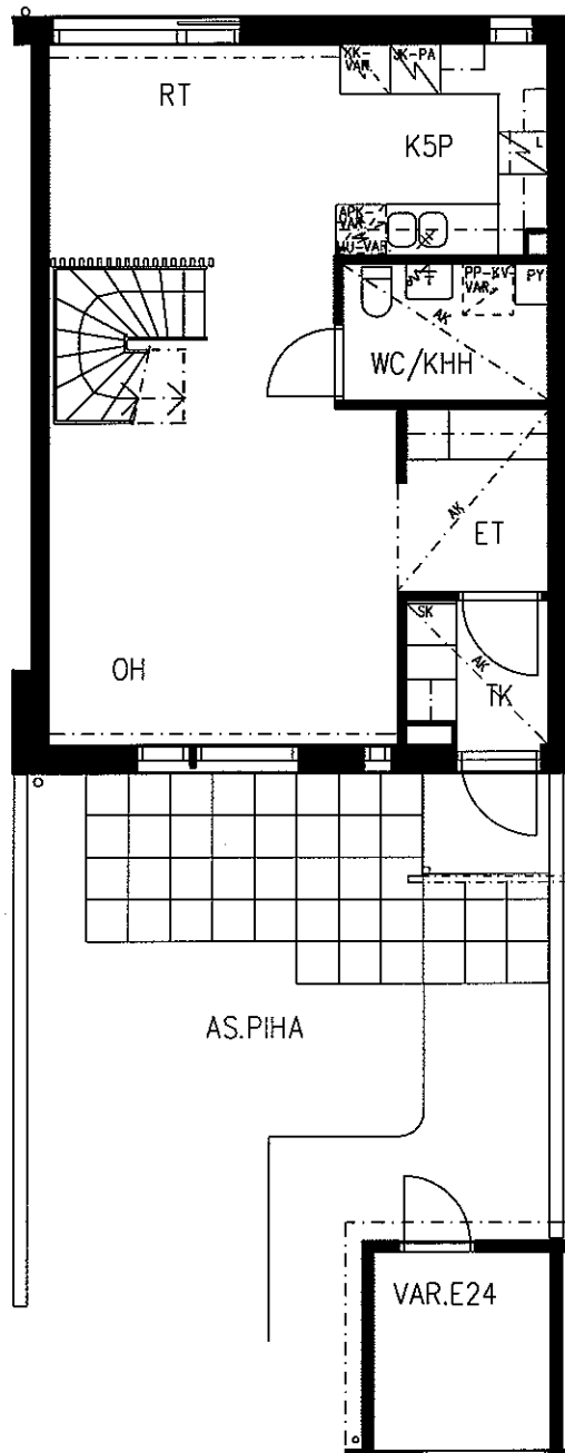
1.KERROS
