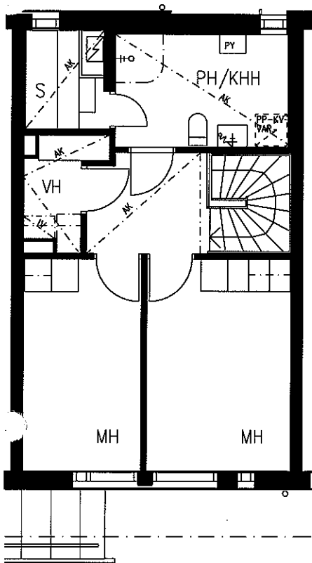
2.KERROS
