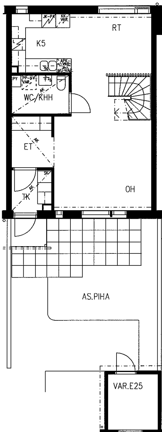
1.KERROS
