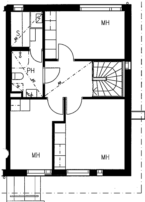
2.KERROS
