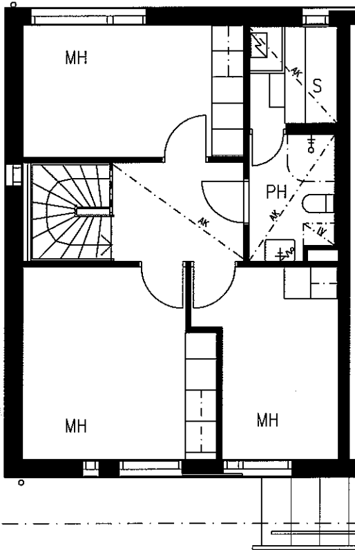
2.KERROS
