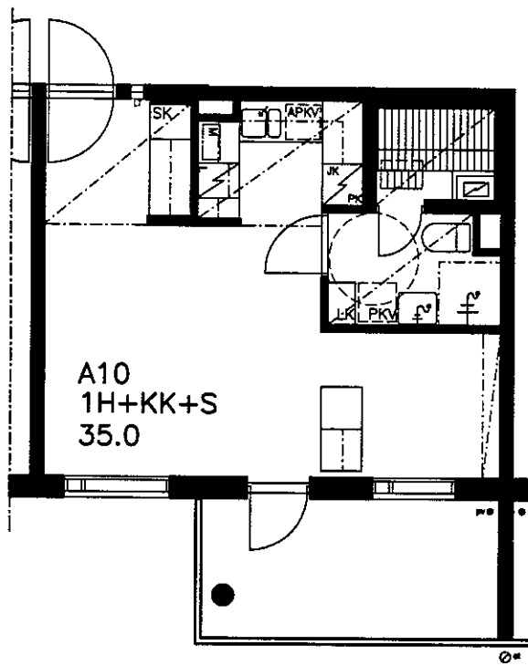
POHJAPIIRUSTUS 1/100
