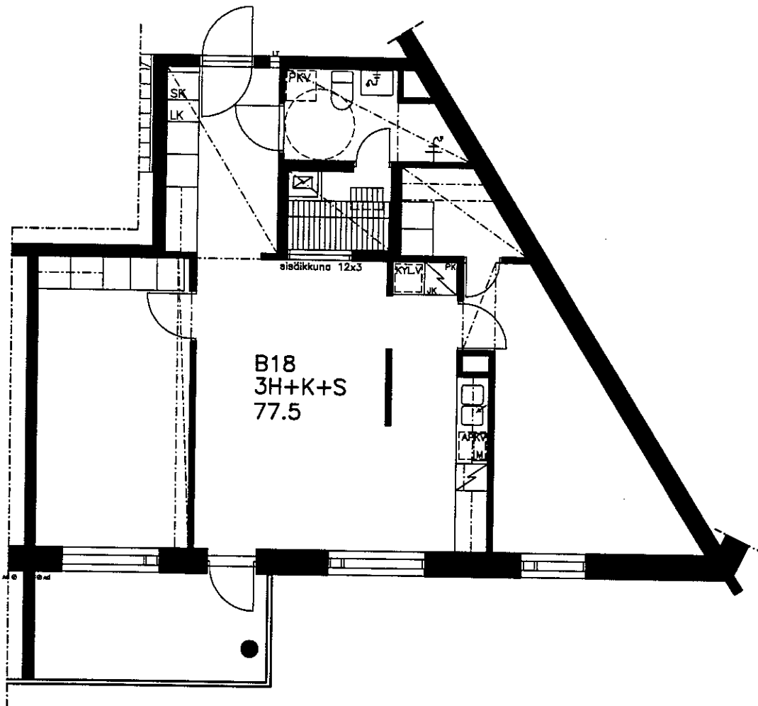
POHJAPIIRUSTUS 1/100
