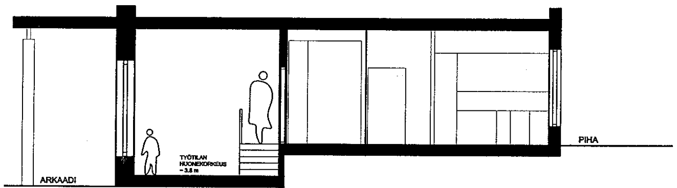
LEIKKAUS B-B
