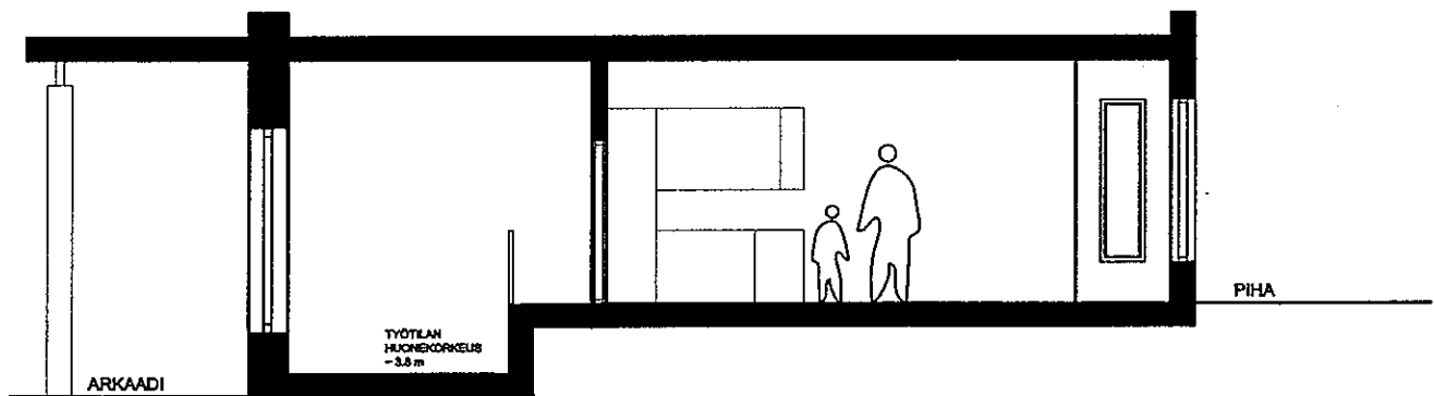
LEIKKAUS C-C
