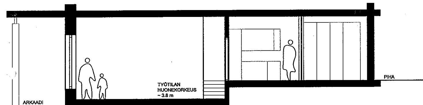
LEIKKAUS A-A
