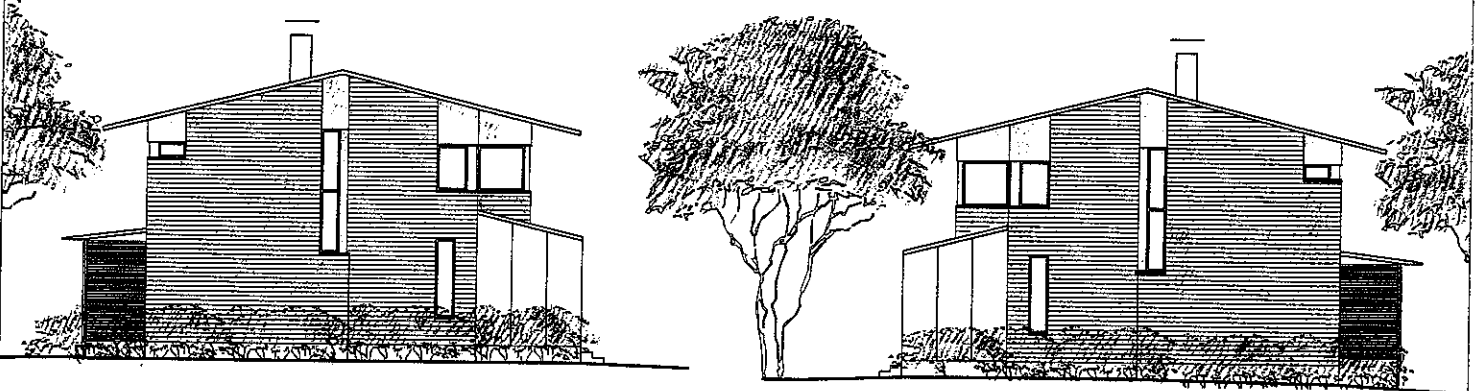
JULKISIVU LUOTEESEEN
